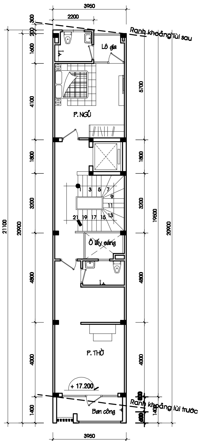
● MẶT BẰNG TẦNG 5 TL : 1/ 100
