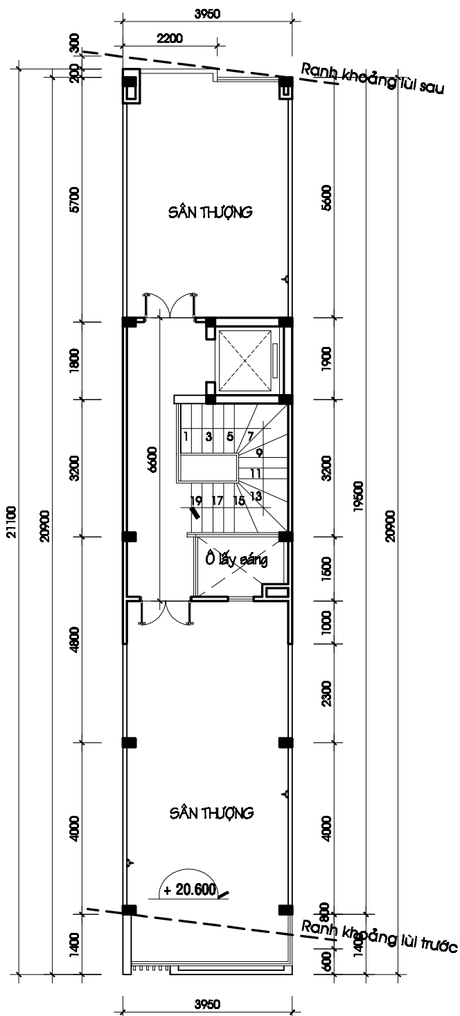
● MẶT BẰNG SÂN THƯỢNG TL : 1/ 100
